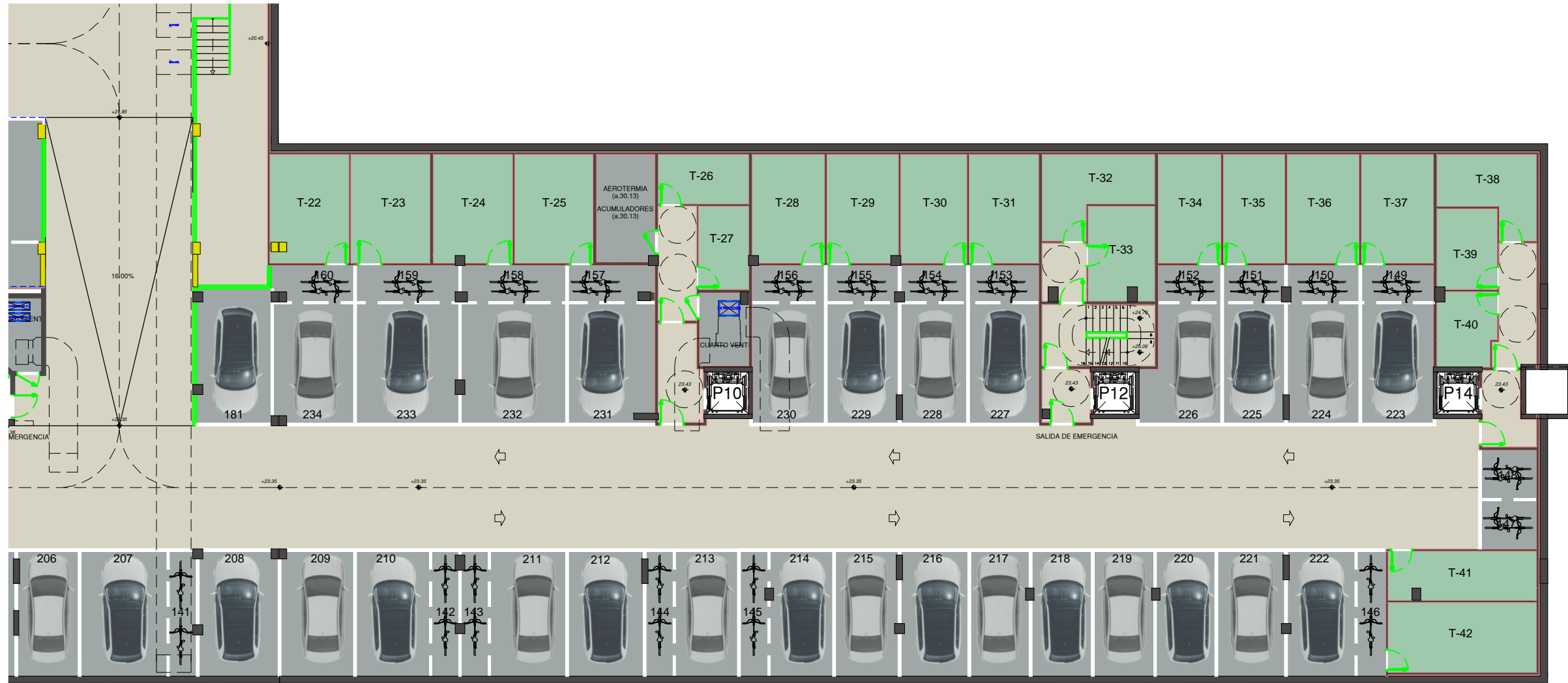
Parcela a.30.12-a.30.14 PLANTA SOTANO -1 Parcela a.30.13 PLANTA SOTANO -2
